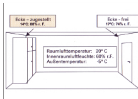
Abb. 3: Auswirkung von Raumecken und Möblierung auf Temperatur und Feuchte. Schimmel entsteht an Wandflächen über 80 % r. F.
